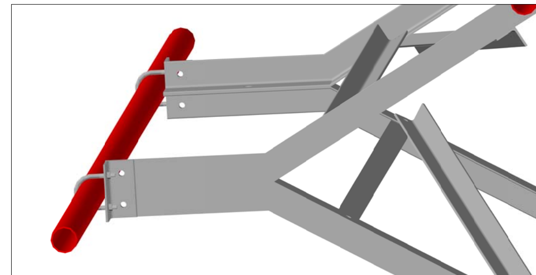
PERSPECTIVA SOPORTE PARA ANTENAS
