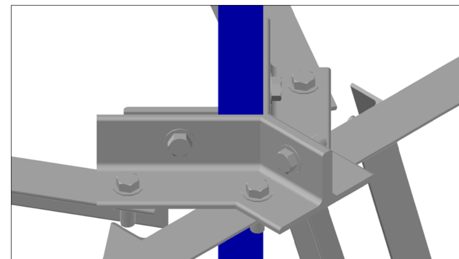
PERSPECTIVA SOPORTE PARA ANTENAS
