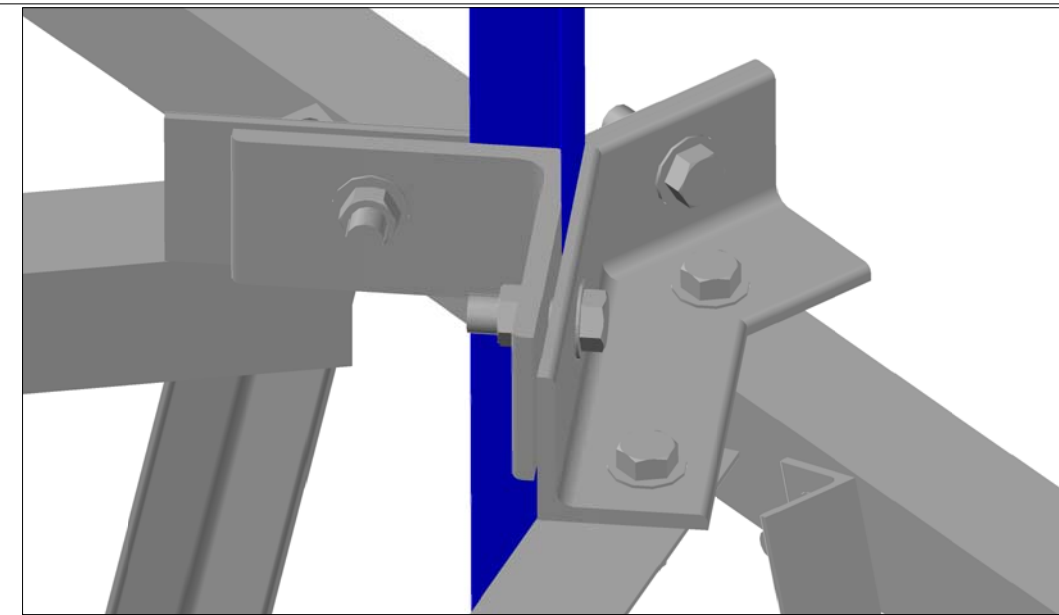
PERSPECTIVA SOPORTE PARA ANTENAS
