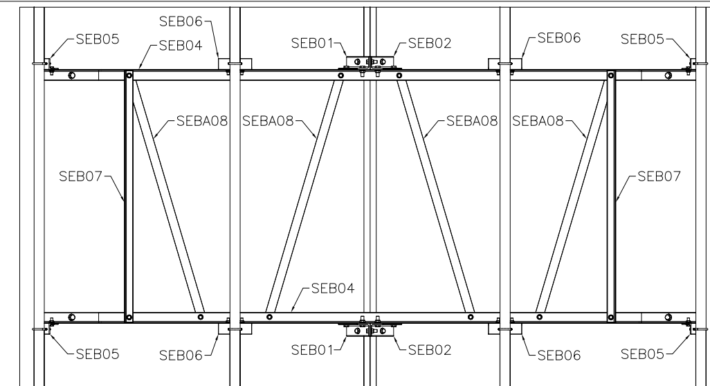
VISTA FRONTAL SOPORTE PARA ANTENAS
