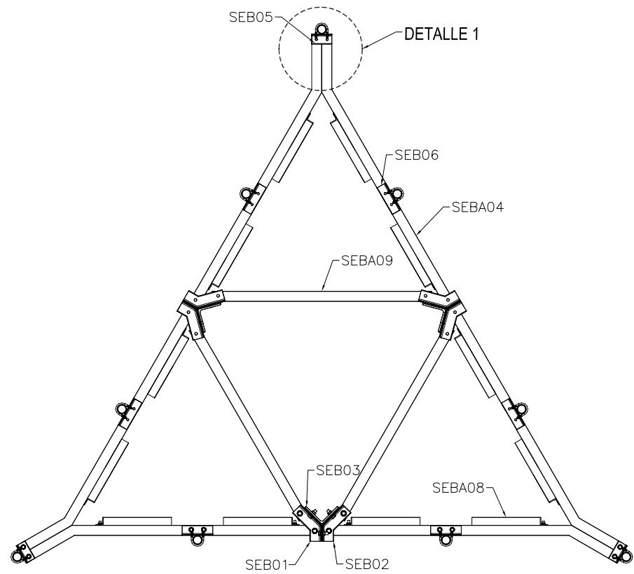
VISTA AEREA SOPORTE PARA ANTENAS
